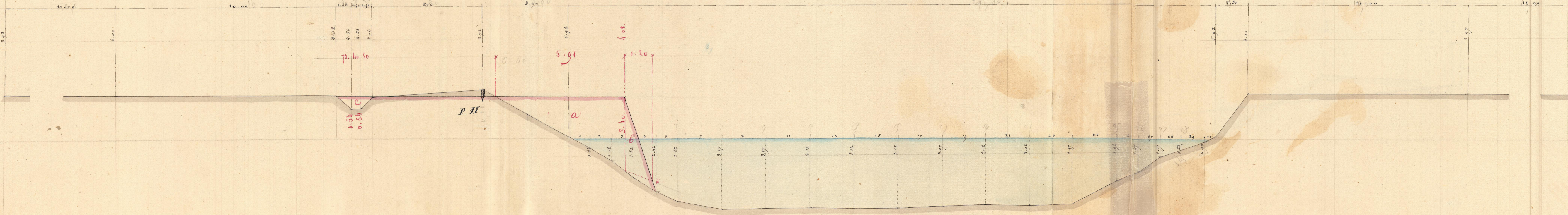
Profil N° 33 à 2200 mètres de l'Cluse (N° 13)
