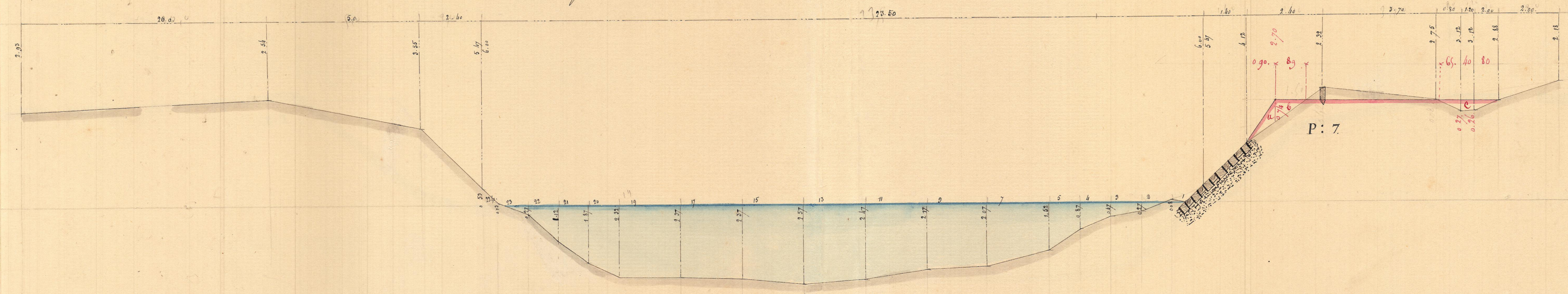
Profil N° 43 à 1400 Metres en Aval de l'Cluse (17)
