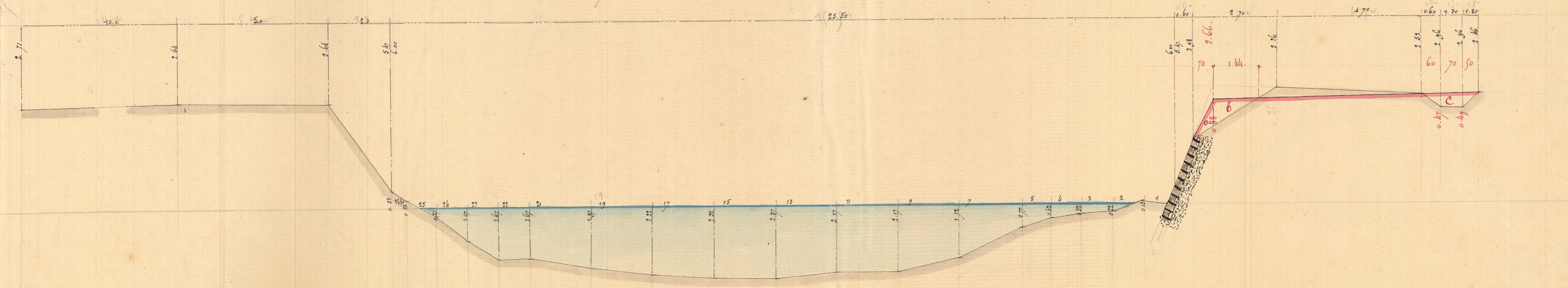
Profil N° 45 à 1500 Metres en Aval de l'Cluse (17)
