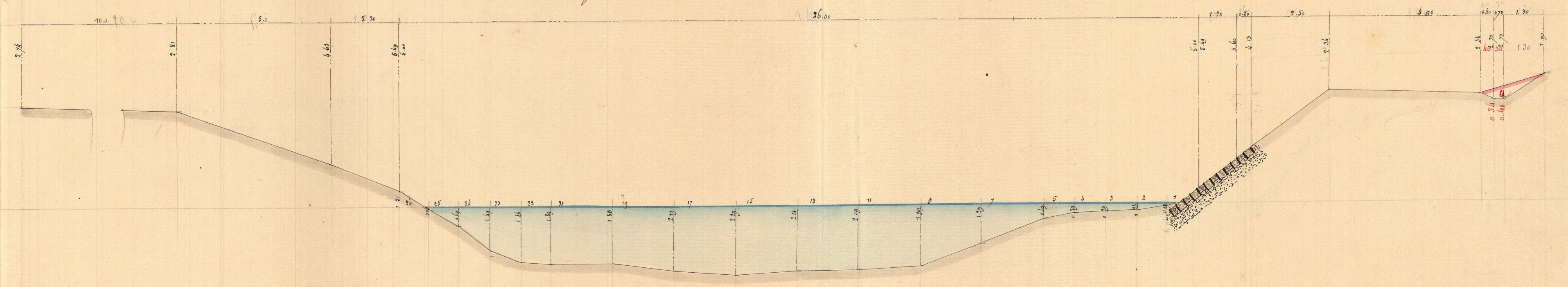
Profil N° 44 à 1485 Metres en Aval de l'Cluse (17)
