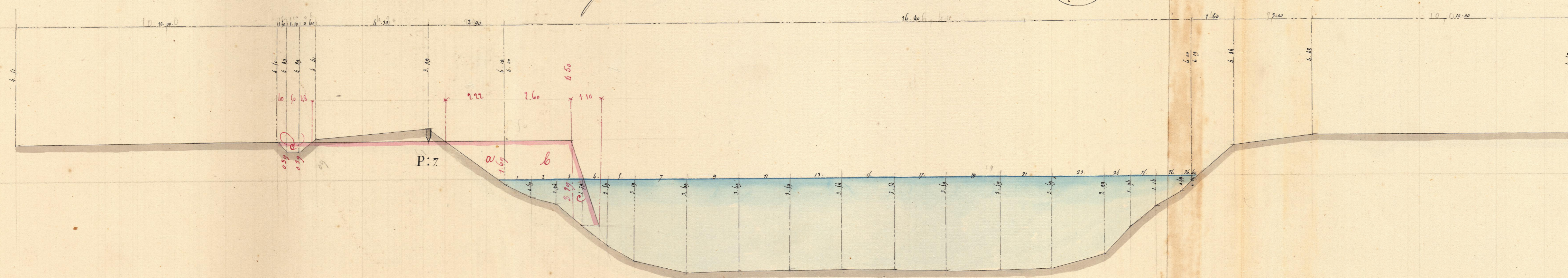
Profil 16° 33 à 1500 metres Det. Cluse (N° 14)
