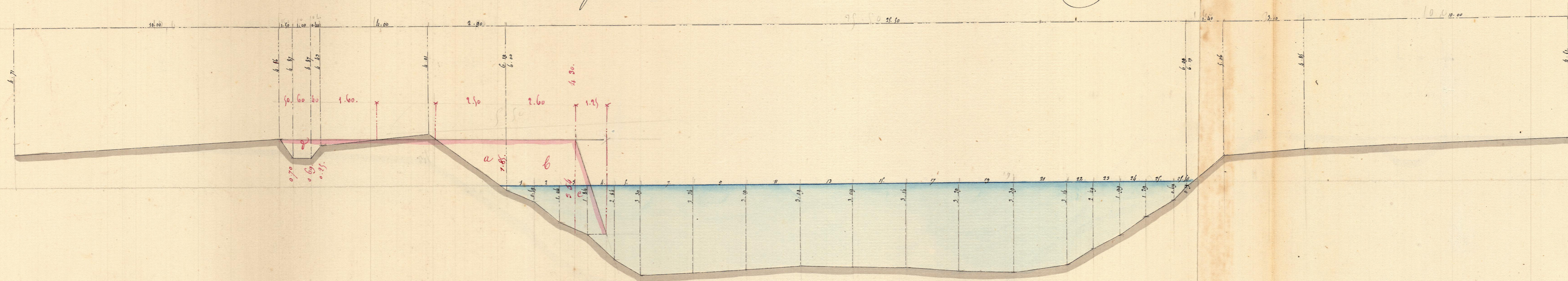
Profil 16° 32 à 1400 metres Det. Cluse (N° 14)
