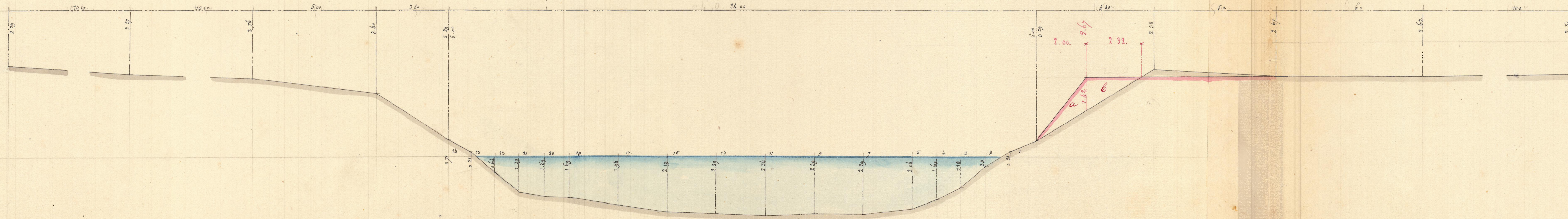
Profil 16° 15 pris à 150 Metres en Amont de l'Cluse (N° 18)
