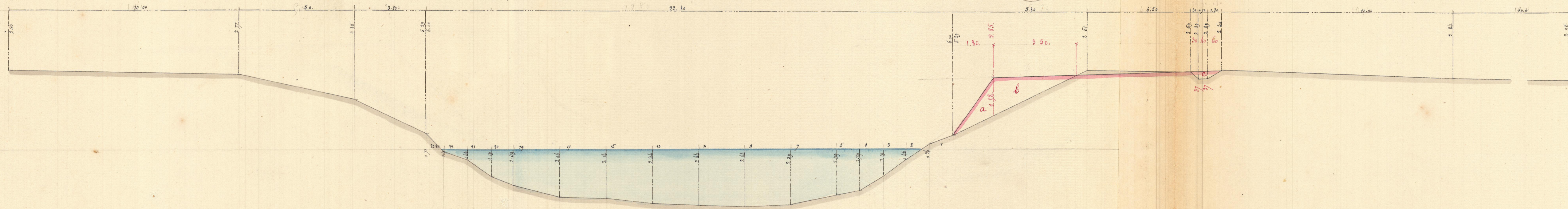
Profil 16° 14 pris à 295 Metres en Amont de l'Cluse (N° 18)
